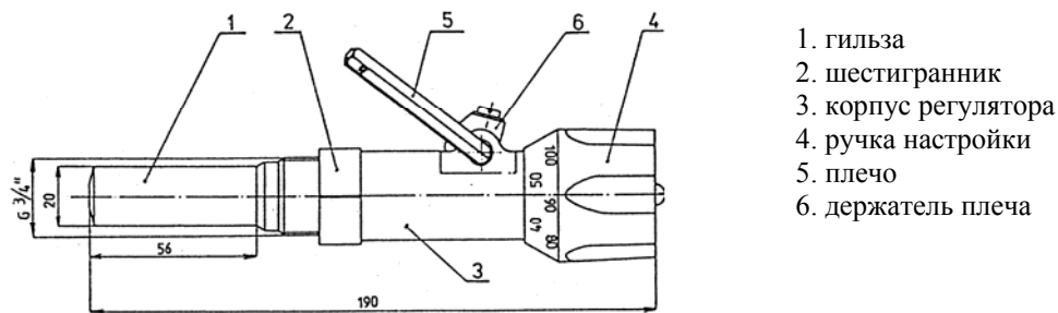
Рис. 1 Температурный регулятор мощности
