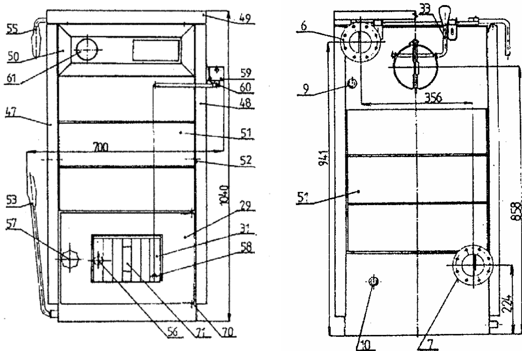
Рис. 5. Отдельные части котла DOR 32
