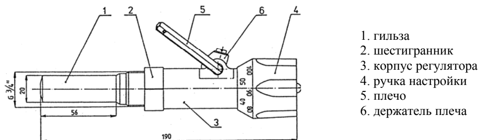
Рис. 1 Температурный регулятор мощности - TRV
