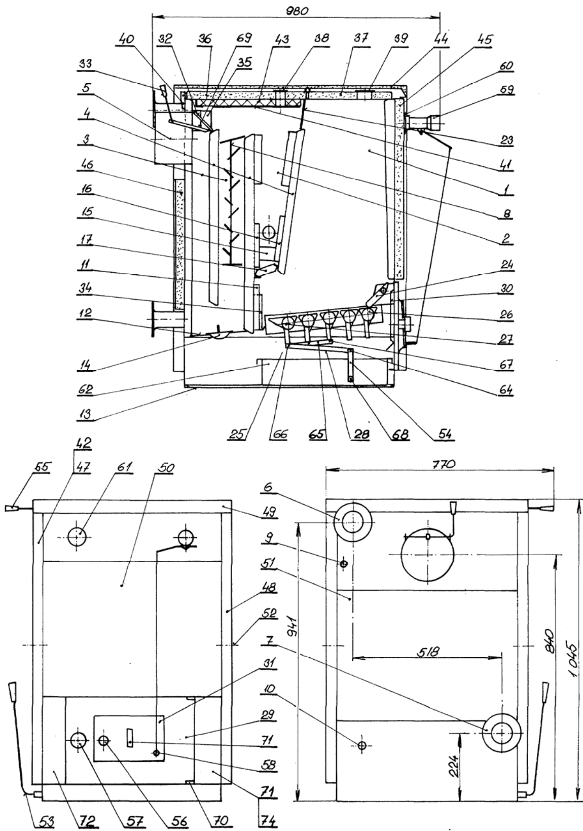
Рис. 2. Котел DOR 45 D
